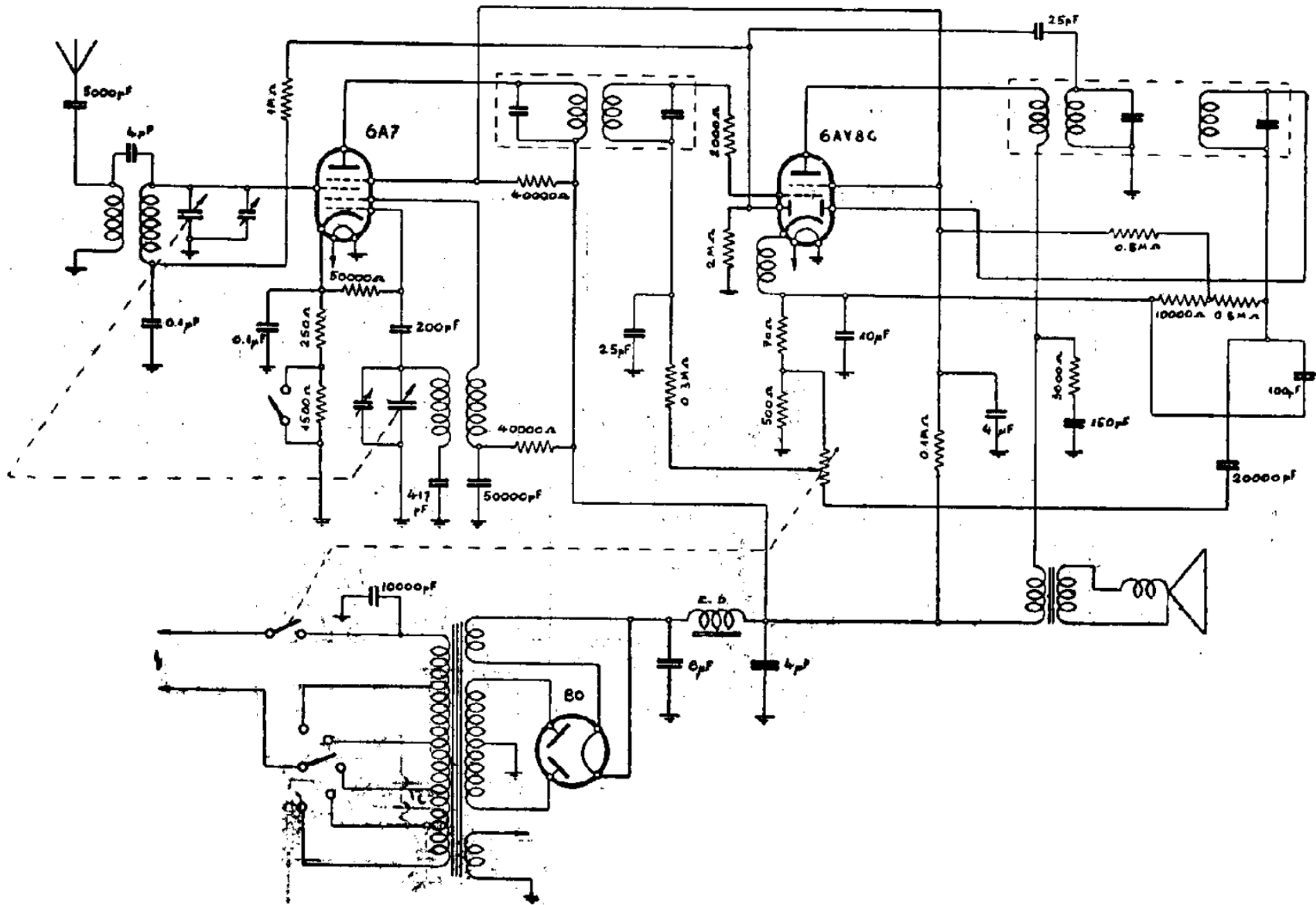
RADIO SAFAR. — Mod. « Roma ». — Media frequenza: 470 kHz. (Questo ricevitore è ampiamente descritto in Moderna Supereterodina, 5ª ediz.)
